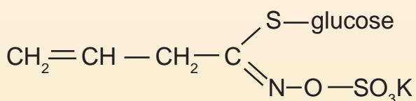
Sinigrin
